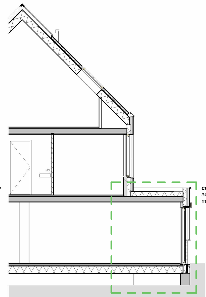
doorsnede
