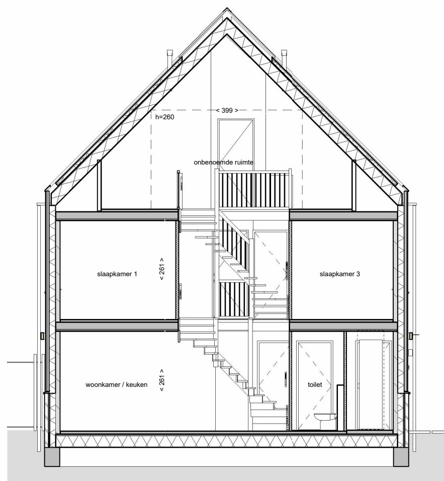
doorsnede
