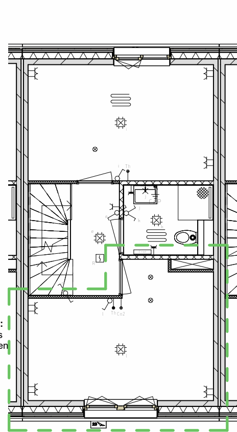
eerste verdieping
