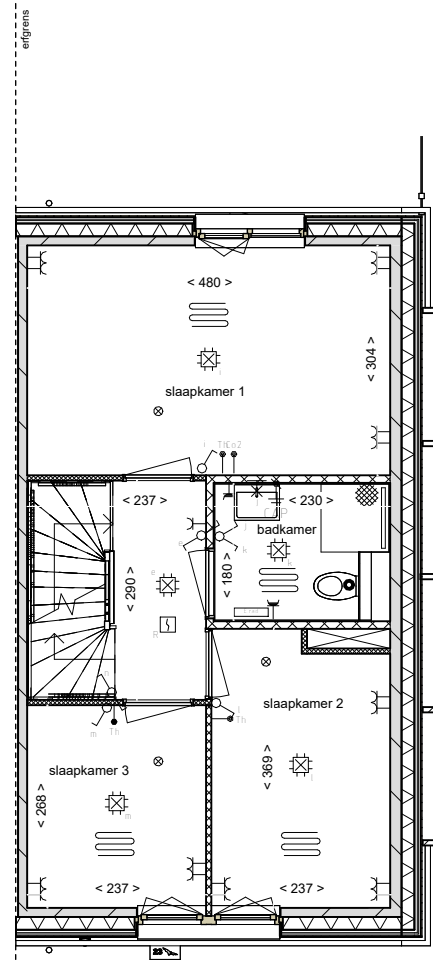
01 eerste verdieping
