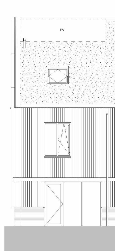
achtergevel
