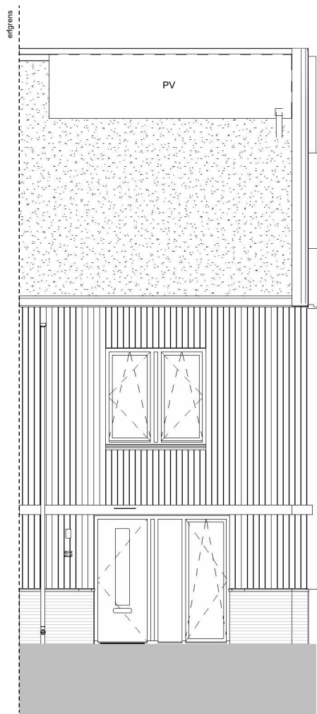
voorgevel
