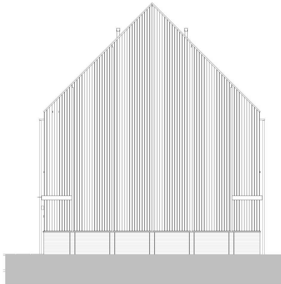
kopgevel
